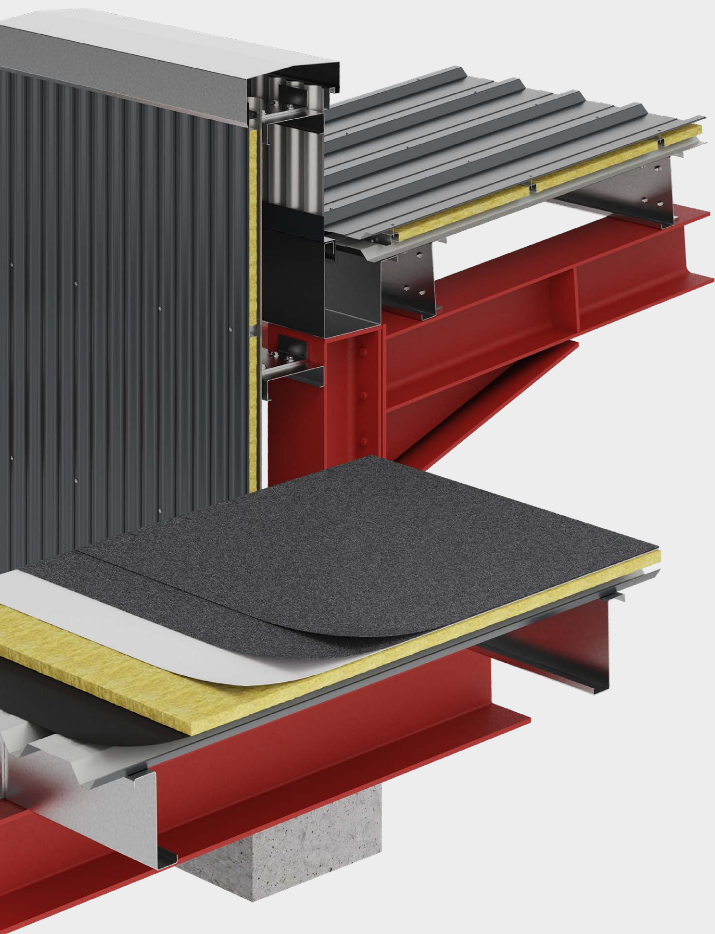
Pormenores construtivos
